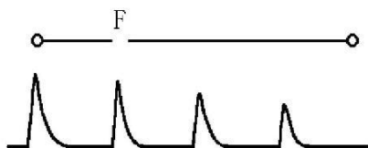
Figure 2A. Forme d'onde de réflexion du défaut de déconnexion
